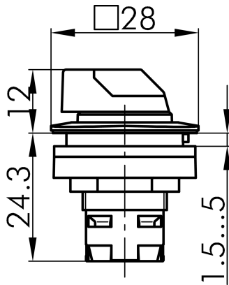
→ Massskizze
