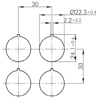
Bohrbild
