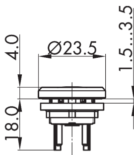
Maßskizze
