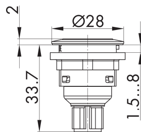
Maßskizze
