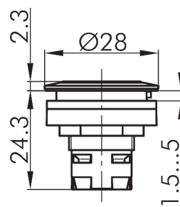
Maßskizze
