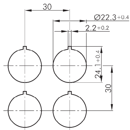
Bohrbild
