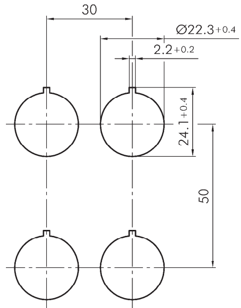
Bohrbild
