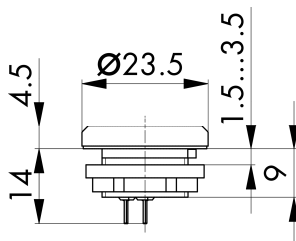
Maßskizze
