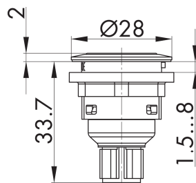
Maßskizze
