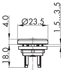
Maßskizze
