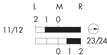
Schaltwegdiagramm
