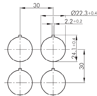
Bohrbild
