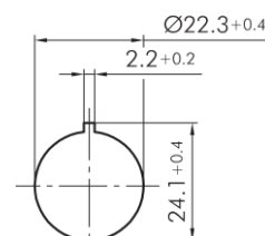
Bohrbild
