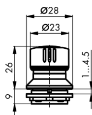
Maßskizze
