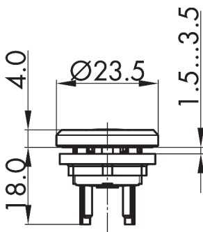
Maßskizze
